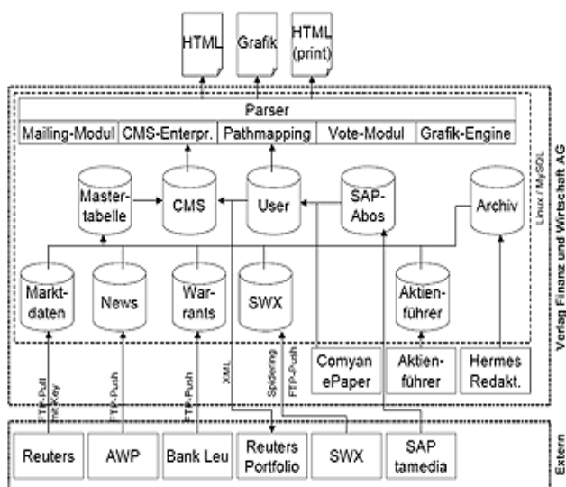
Datenkonzept / -architektur
